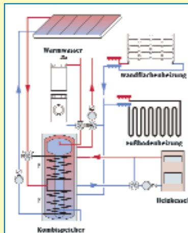
Kombianlage
