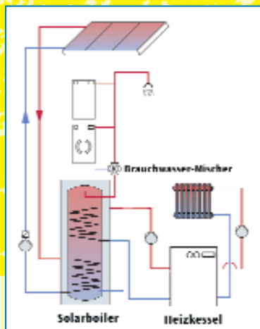
Brauchwasseranlage
